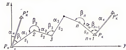
Рис. 1. Полигонометрический ход.
